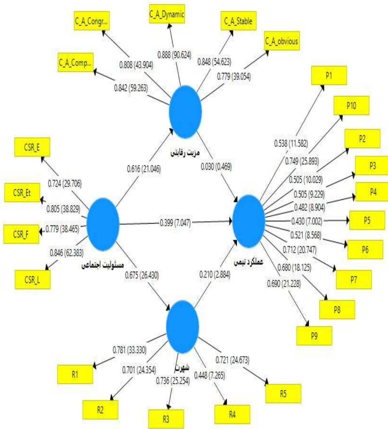
شکل ۲. خروجی نرم افزار Smart PLS 3
