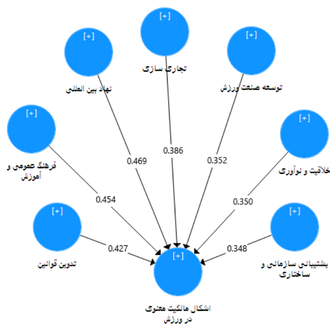
شکل ۱- مدل خروجی تحقیق در حالت ضریب مسیر
